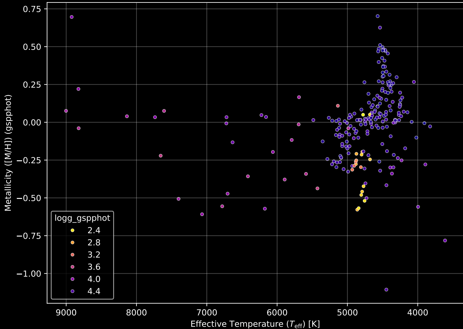
APOGEE DR17 Field: [M67-S] Stellar Population Parameters (n= 229)
